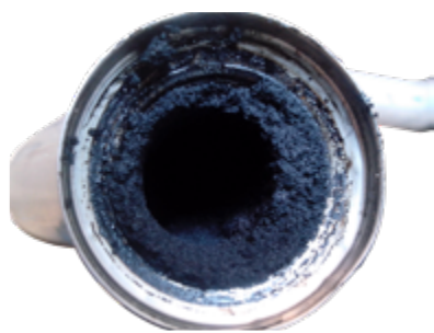
Verschmutztes Volkswagen 1.6 EGR-Rohr nach 86.000 km!
